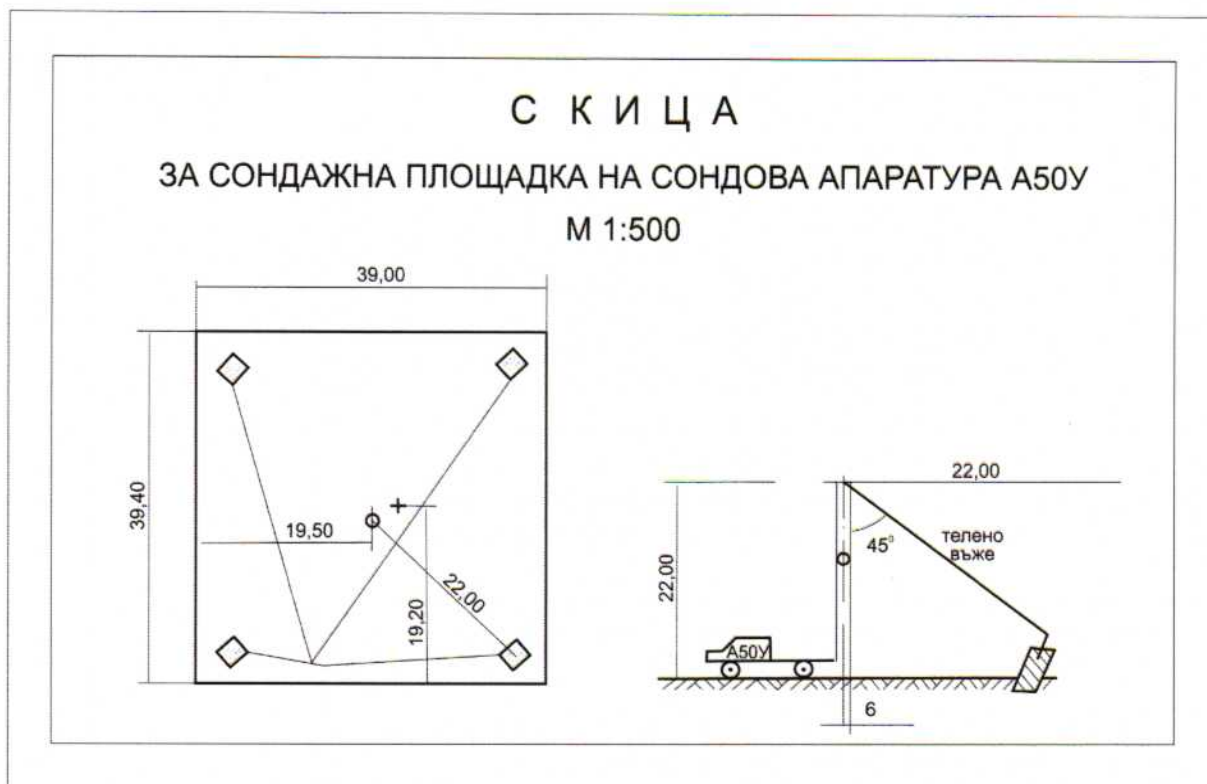
Фиг. 1. Скица за сондажна площадка на сондова апаратура A50Y
